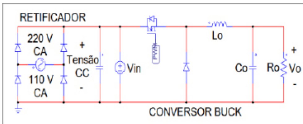
Figura 1 - Circuito conversor Buck
