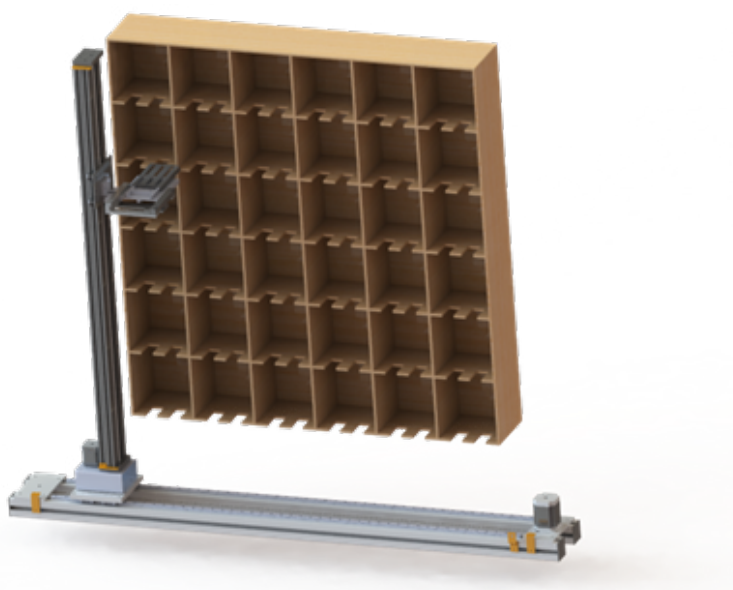
Figura 2 - Sistema AS/R
