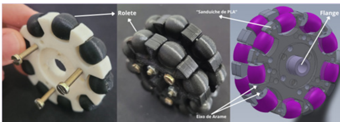
Figura 1 - Roda omnidirecional modelada e desenvolvida
