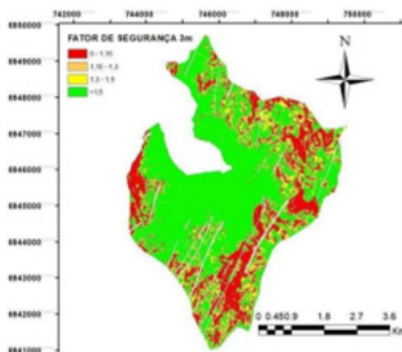
Figura 5 - Mapa do Fator de segurança de 3 metro da Bacia Hidrográfica do Itacorubi
