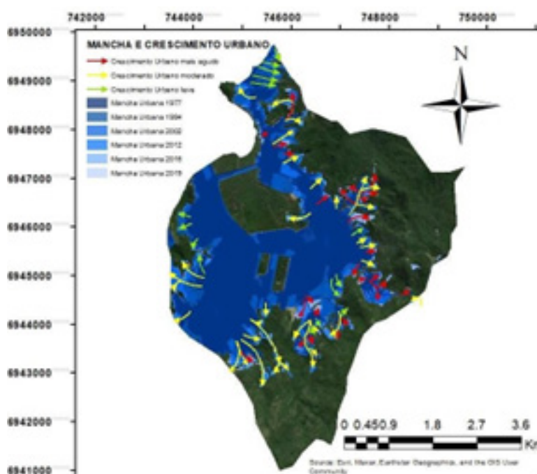
Figura 8 - Mapa da mancha e crescimento urbano da Bacia Hidrográfica do Itacorubi
