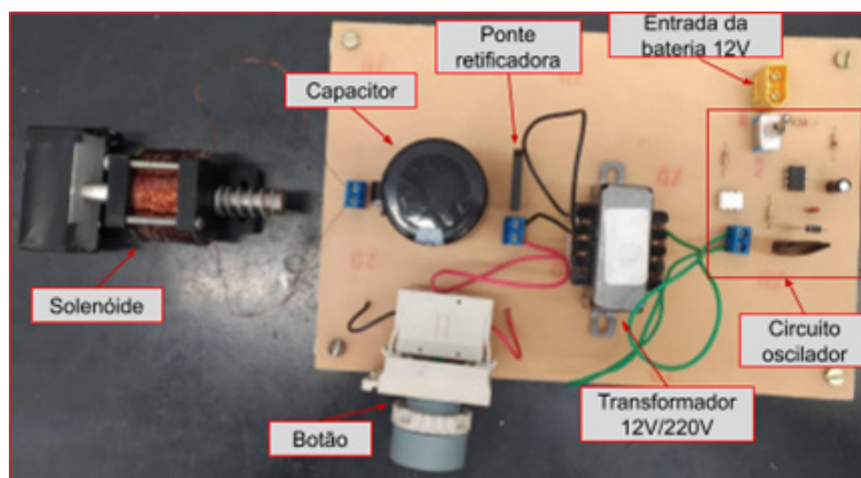
Figura 2 - Sistema do Kicker
