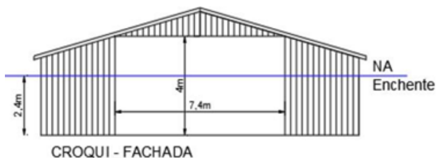
Figura 7 - Exemplo de croqui elaborado a partir das vistorias
