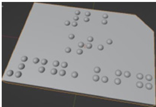
Figura 3 - Face superior do modelo do elemento titânio no software Blender
