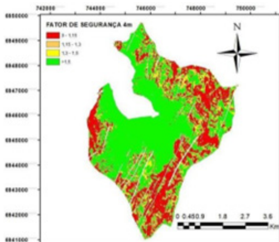
Figura 6 - Mapa do Fator de segurança de 4 metro da Bacia Hidrográfica do Itacorubi
