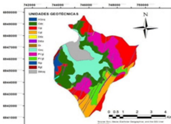
Figura 2 - Mapa de unidades geotécnicas da Bacia Hidrográfica do Itacorubi
