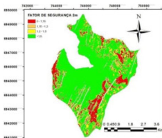
Figura 4 - Mapa do Fator de segurança de 2 metro da Bacia Hidrográfica do Itacorubi
