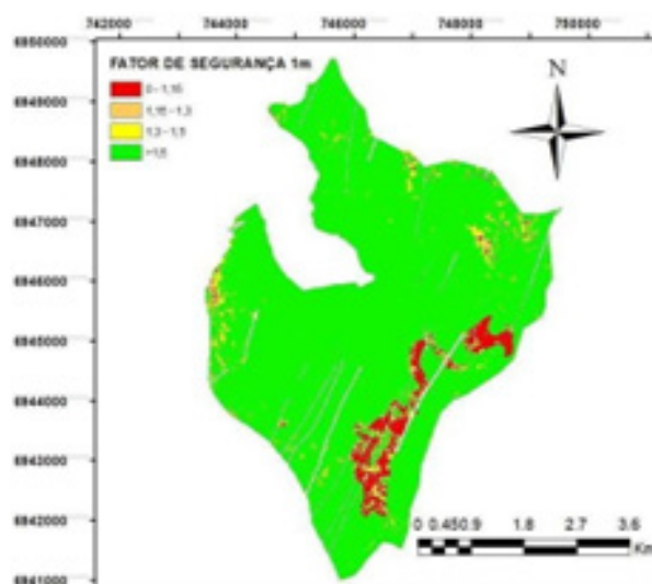
Figura 3 - Mapa do Fator de segurança de 1 metro da Bacia Hidrográfica do Itacorubi
