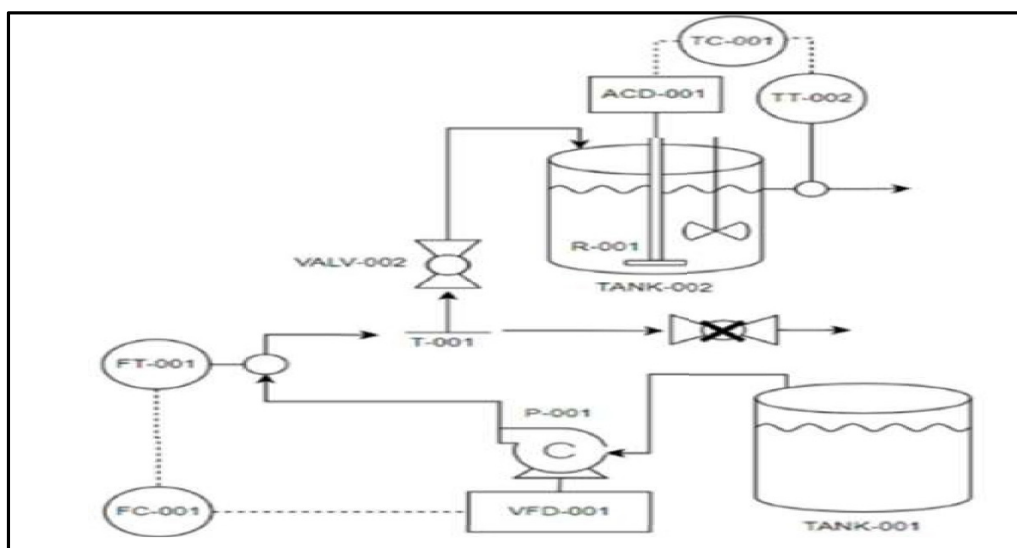
Figura 1 - Representação Esquemática do PCA
