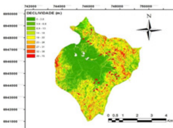
Figura 1 - Mapa de declividade da Bacia Hidrográfica do Itacorubi
